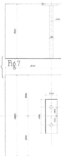
je 2 Stück zur Lagerung der Vorgelegewelle.
