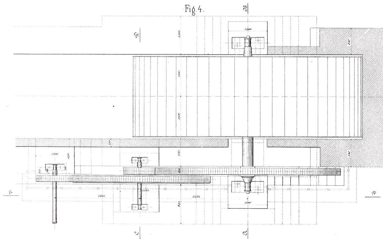
je 2 Stück zur Lagerung der Wasserradwelle.
