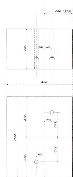
je 2 Stück zur Lagerung der Wasserradwelle.
