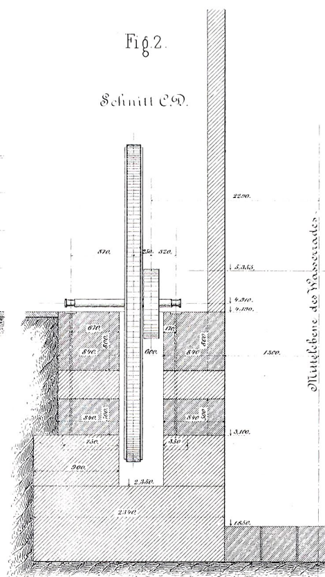
je 2 Stück zur Lagerung der Wasserradwelle.
