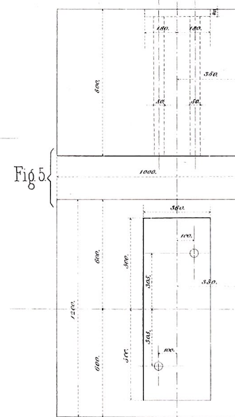
je 2 Stück zur Lagerung der Wasserradwelle.
